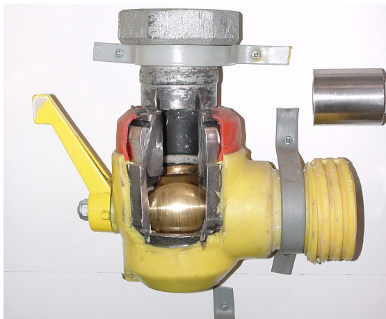
Hauptabsperreinrichtung (Darstellung Teilaufschnitt)
