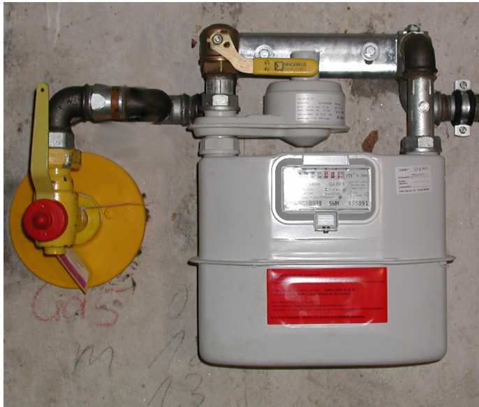
Einzelspartenanschluss mit Gaszähler und Zählerregler
