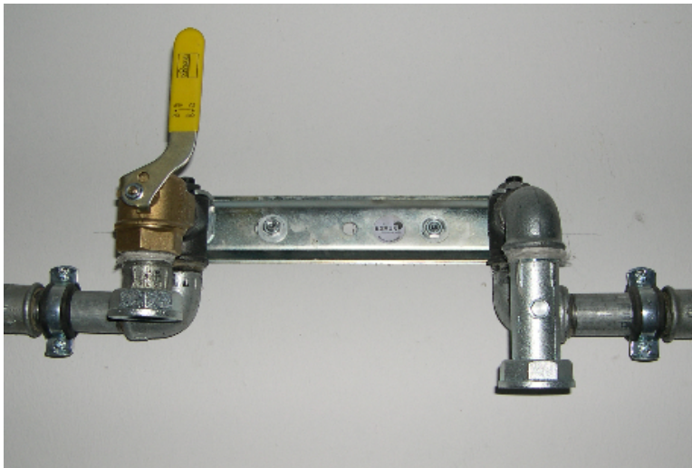
Gaszähleranschlussplatte
