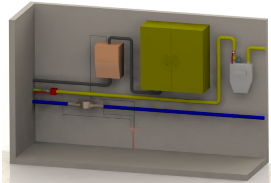
Beispiel: Hausanschlusswand
